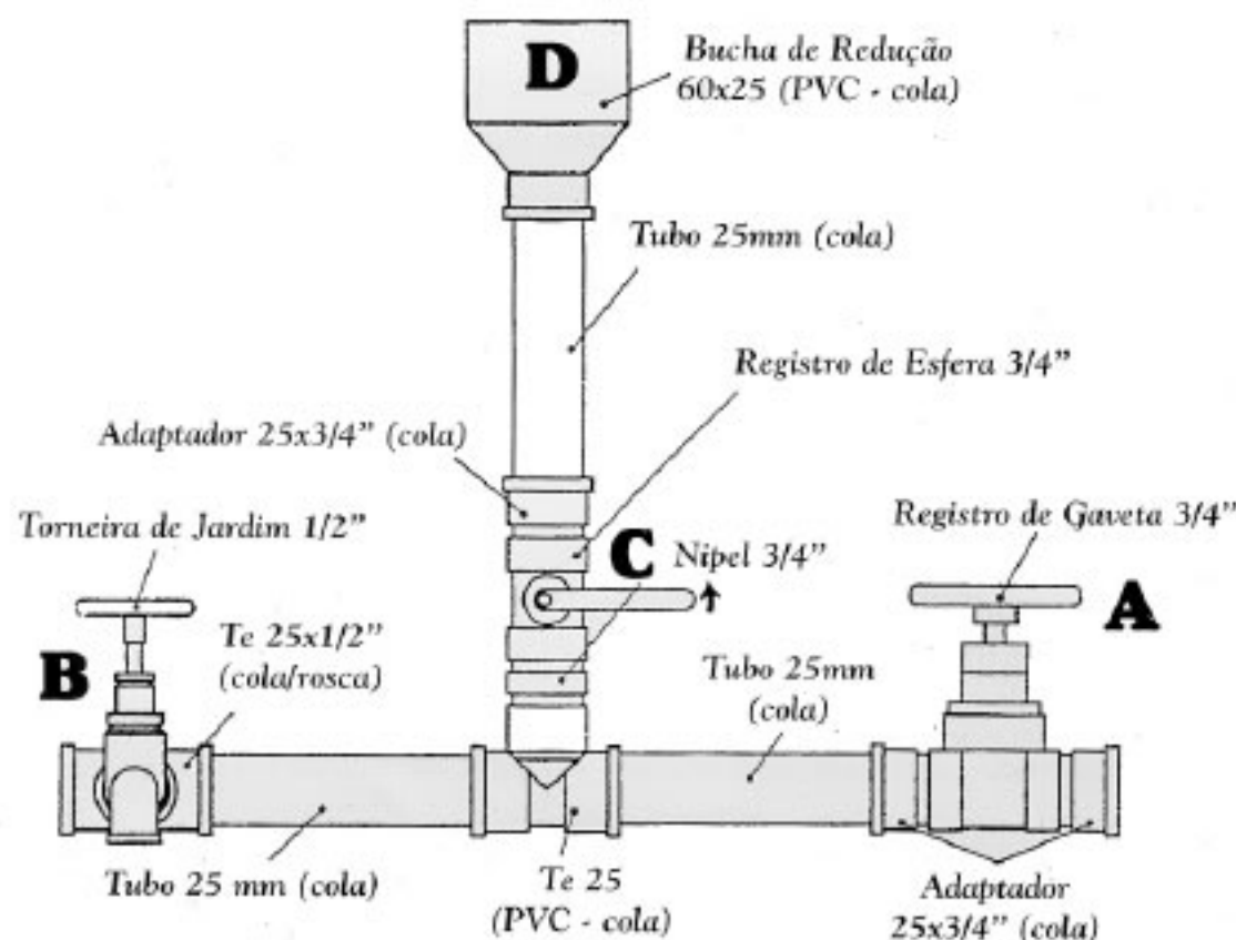
Figura 2 - Esquema de montagem do clorador de água.
